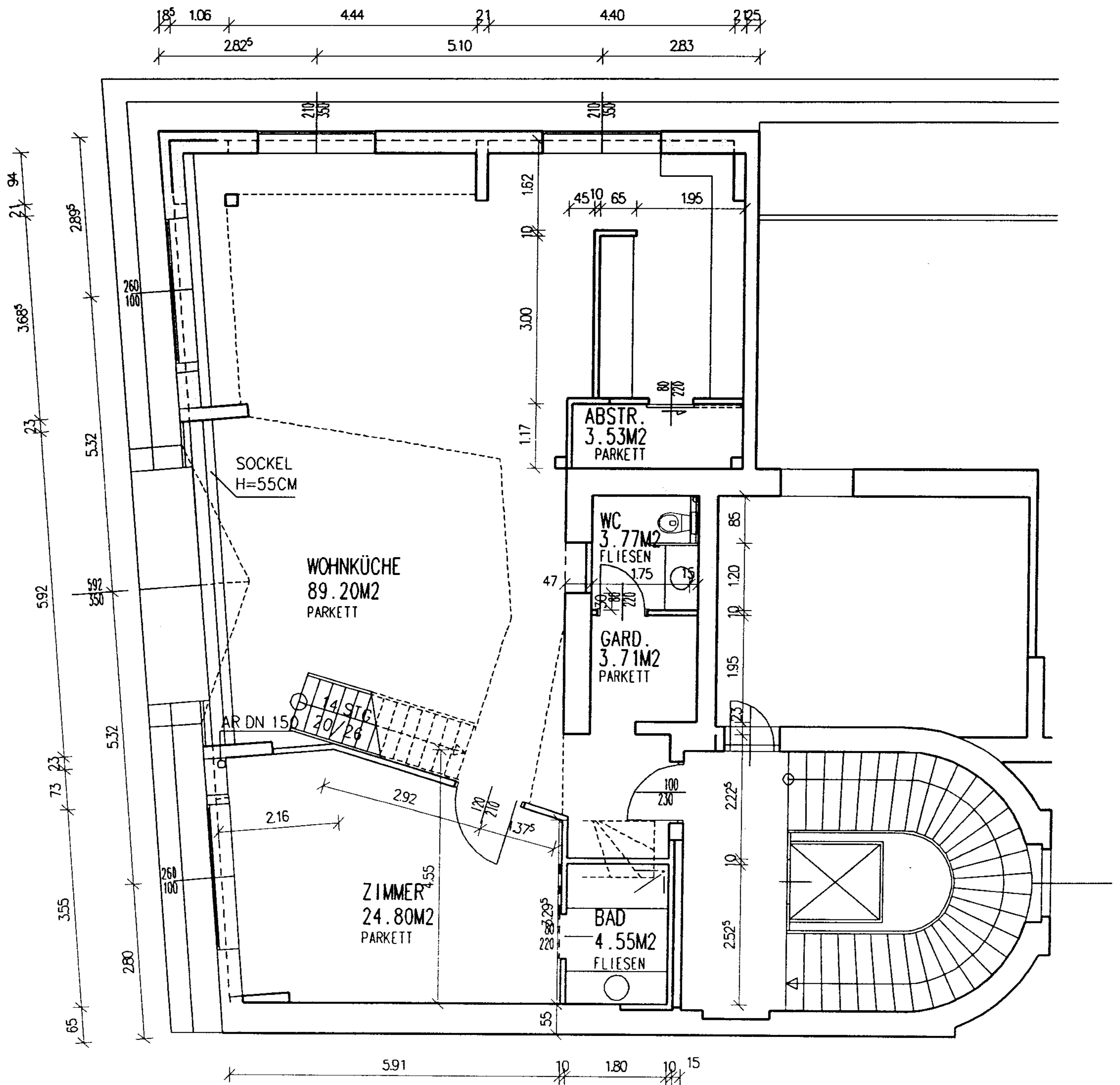
GRUNDRISS DACHGESCHOSS
