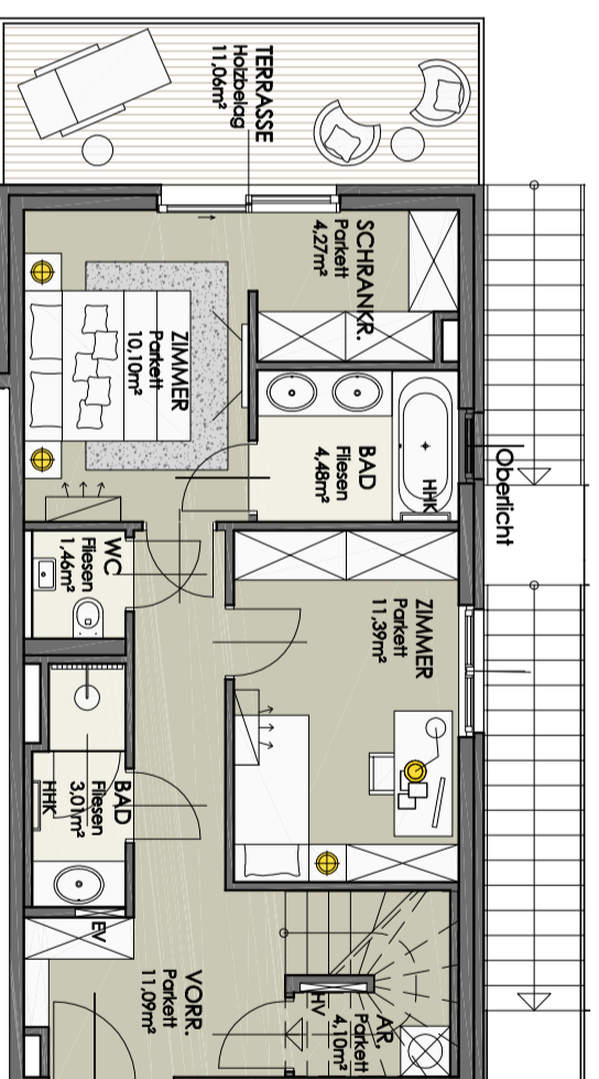
2. OBERGESCHOSS
